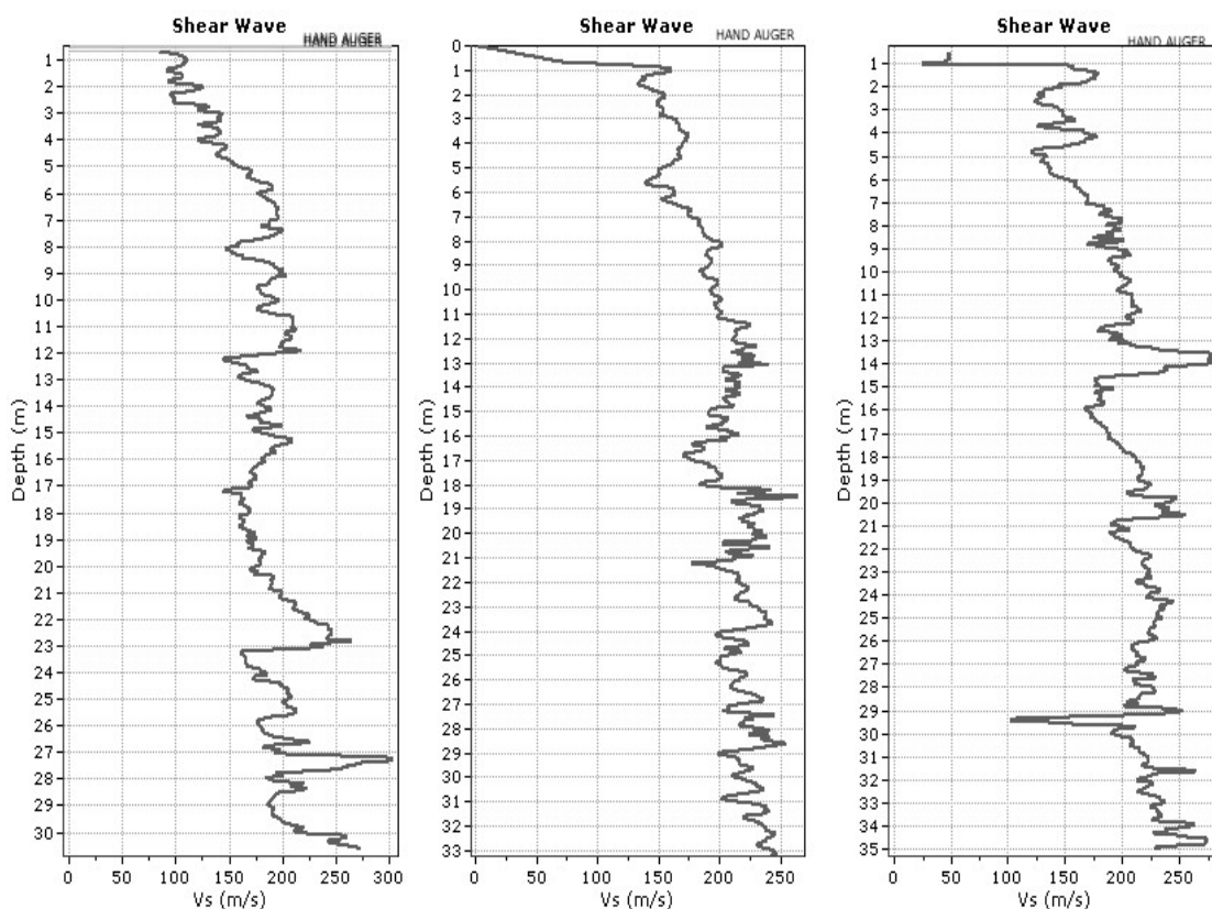
Figura 3.3 – Distribuzione delle Vs ricavate dagli esiti delle prove CPTU d'archivio RER: U501 per l'area “ex Zuccherificio; U502 e U503 per la frazione Massumatico
