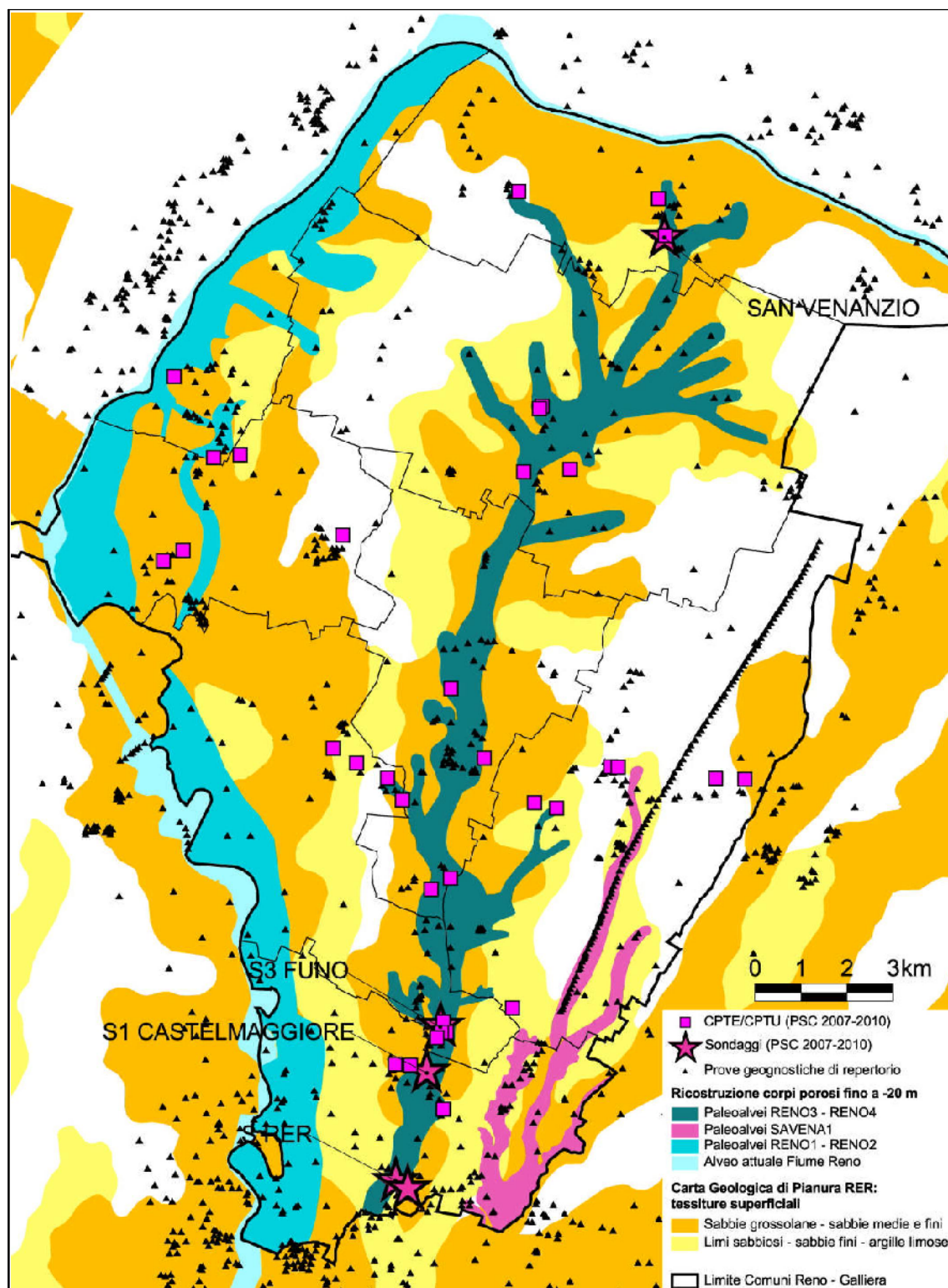
Figura 3.1 – Ricostruzione dei corpi porosi fino a 20 metri di profondità
