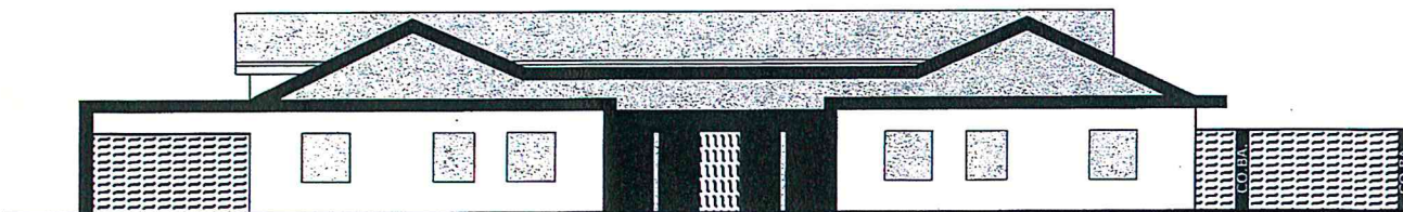
PROSPETTO OVEST (da via 2 giugno)
