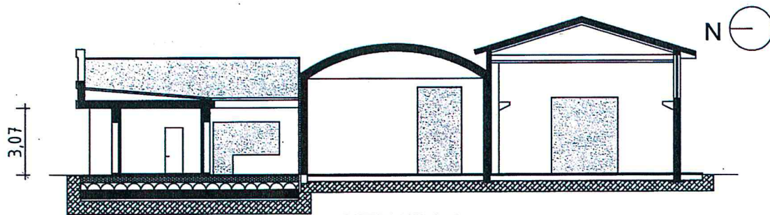
SEZIONE A-A
