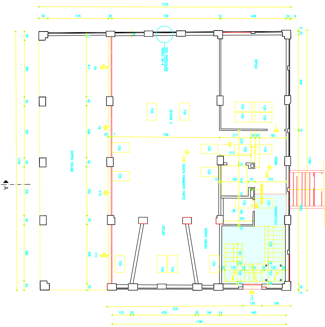
PIANTA PIANO PRIMO (FINITURA AL GREZZO)
