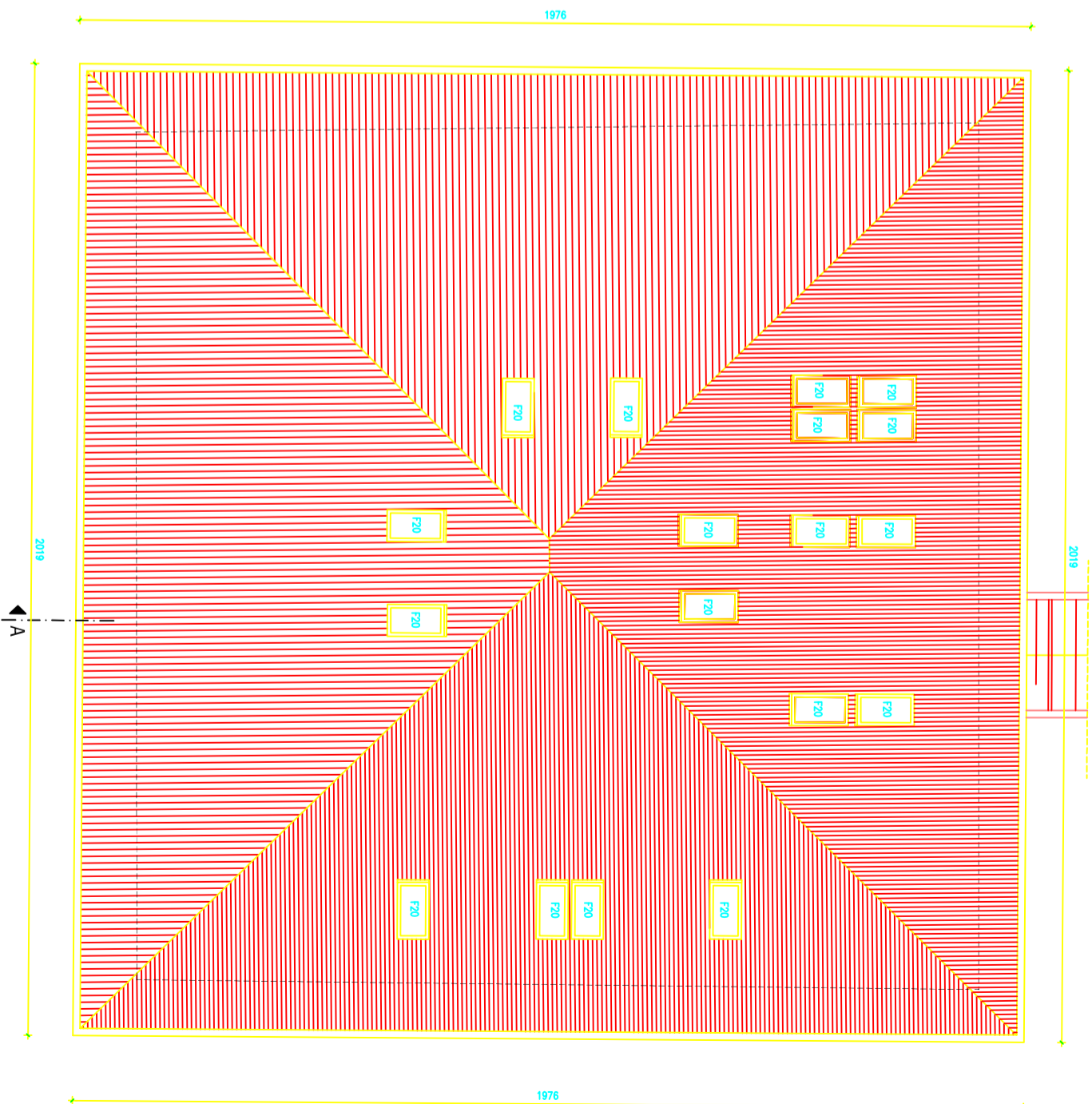
PIANTA PIANO COPERTURA
