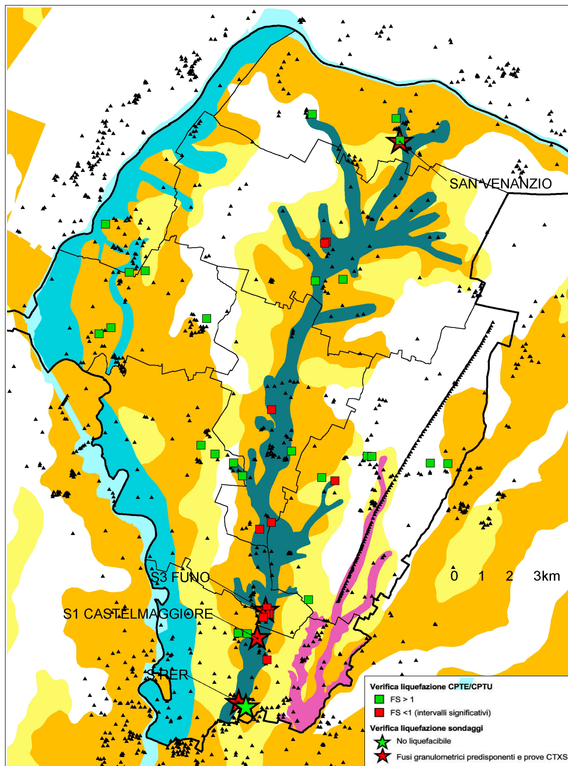
Figura 3.2 - Sintesi delle verifiche di di liquefazione espletate per i PSC dei Comuni dell'Unione Reno-Galliera (prove CPTE/CPTU e prove triassiali cicliche di laboratorio)
