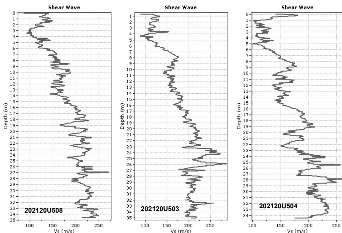
Figura 3.3bis – Distribuzione delle Vs ricavate dagli esiti delle prove CPTU d'archivio RER
